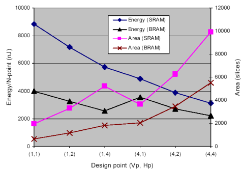
(그림 4) N=256 일 때 다양한 디자인에 대한 에너지와 면적의 추정치
